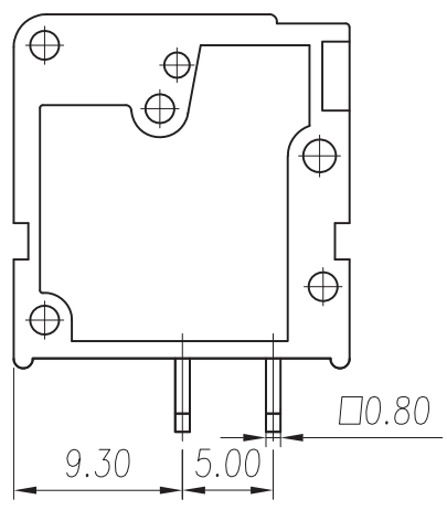
p.c.b. layout
