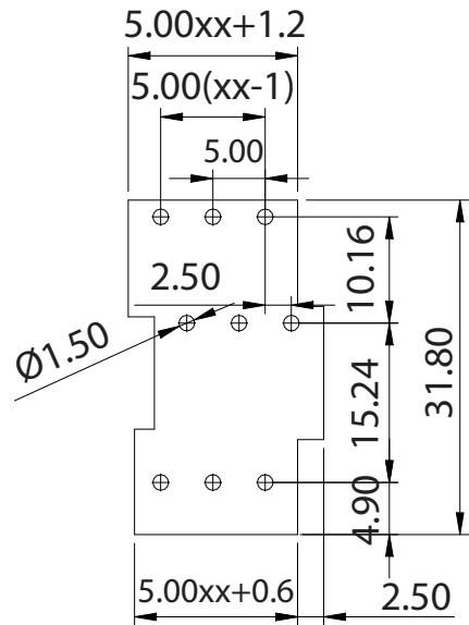
p.c.b. layout
